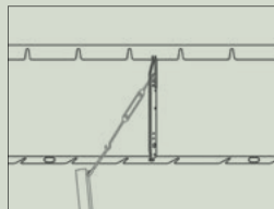
STAP 4B - BEVESTIG MET VERSTEVIGINGSELEMENT
